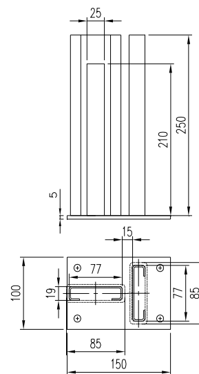
Abb. 2 Befestigung mit horizontalen Bügeln aus Edelstahl
