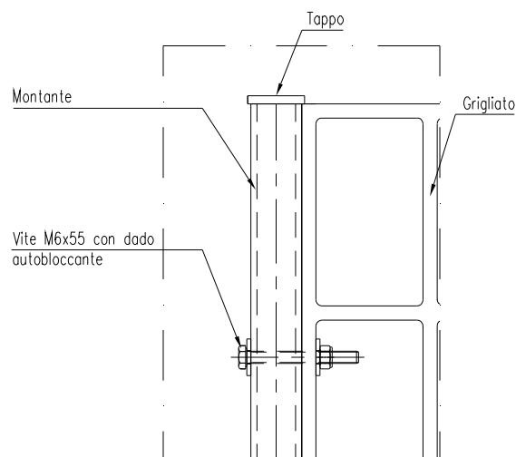
Abb. 4 Befestigung des Gitterrosts am Pfosten
