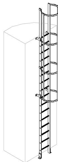
Fig. 3 Leiter mit mehreren Halterungen
