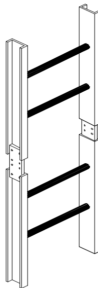
VERBINDUNG ZU LEITERTYP 3 GFK-Platte 230x72 mm, Stärke 15 mm E23 pultrudiert
