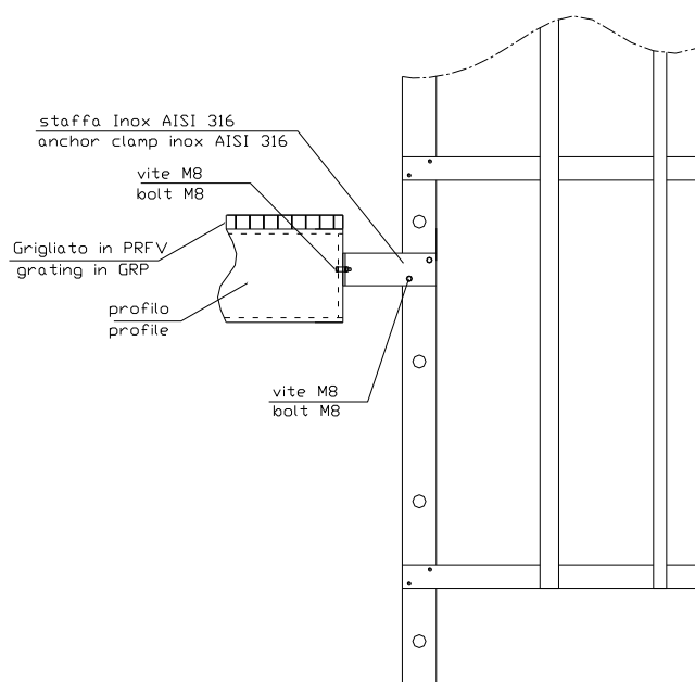
Fig. 5 Befestigung der Leiter an GFK-Laufsteg
