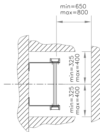
Schnittansicht einer Leiter ohne Rückenschutz
